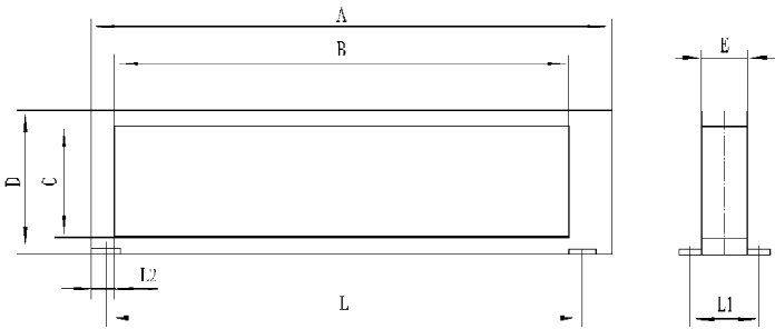
JYG- B 金属探测仪外形图
