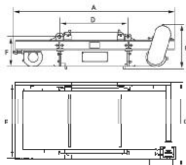
外形尺寸图
