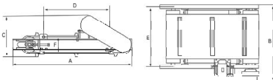
外形尺寸图
