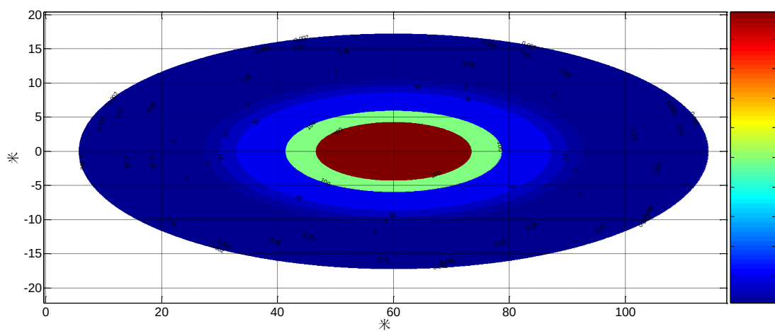
图 5.4-45 生产废水酚污染物在瞬时渗漏运移 3000 天后的浓度变化平面图
