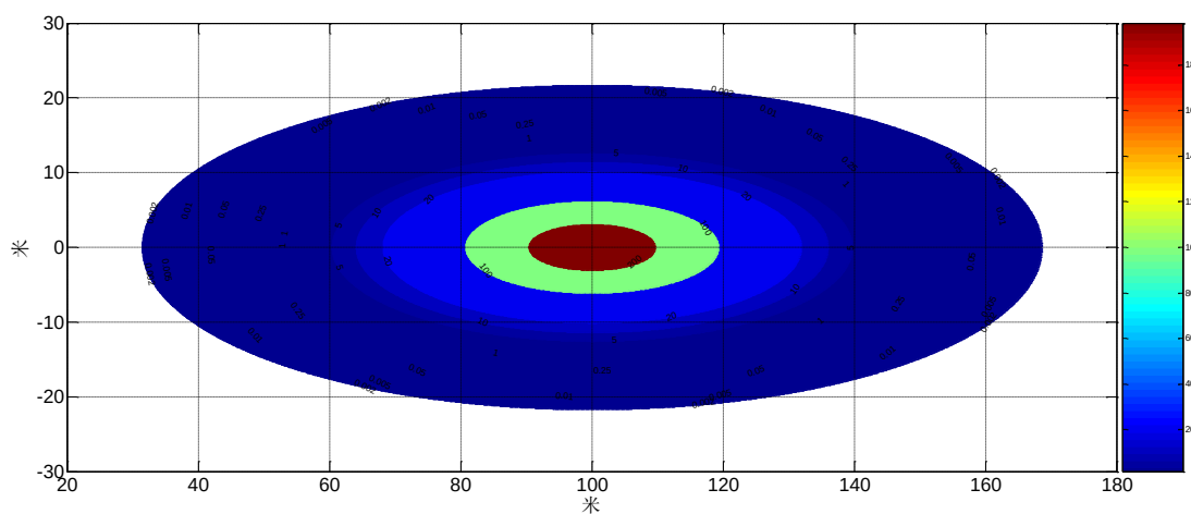
图 5.4-46 生产废水酚污染物在瞬时渗漏运移 5000 天后的浓度变化平面图
