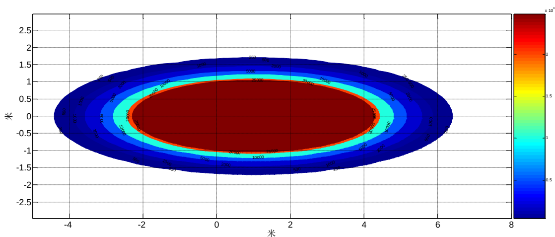
图 5.4-47 生产废水硫酸盐污染物在瞬时渗漏运移 50 天后的浓度变化平面图
