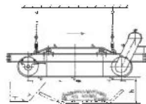
安装示意图（水平式）
