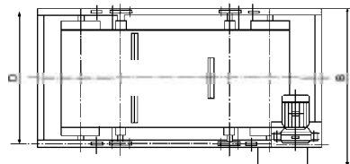
外形尺寸图
